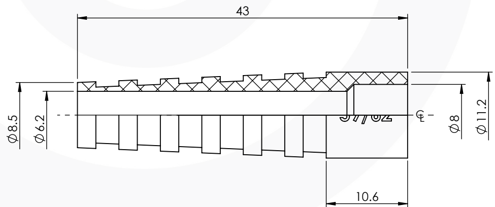
SECTION A-A SCALE 2 : 1
