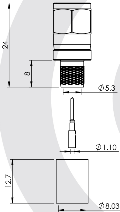
HEX 11 A/F
